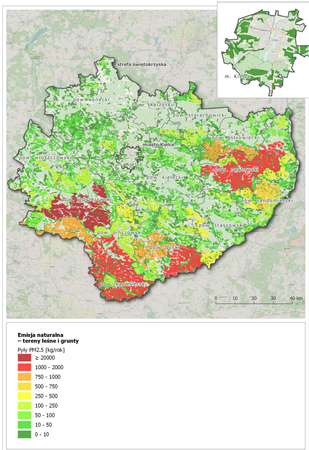
Rysunek 44. Emisja naturalna pyłu PM 2,5 z terenów leśnych i gruntów 109
