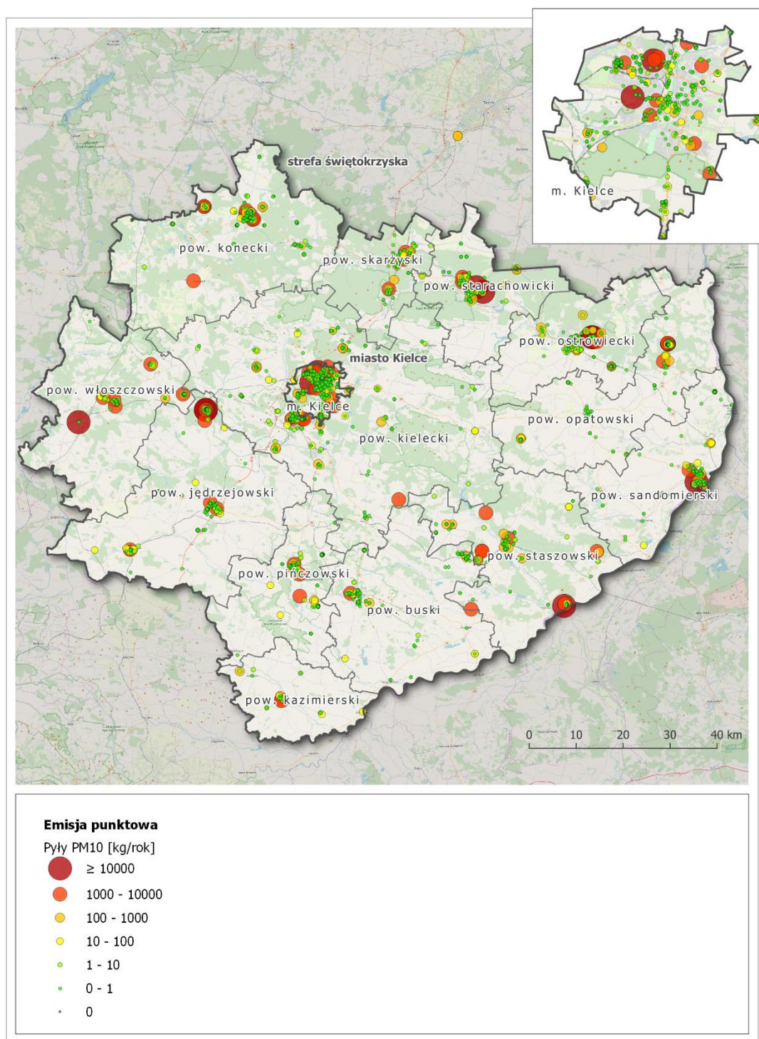
Rysunek 31. Emisja pyłu PM10 ze źródeł przemysłowych i energetycznych 96
