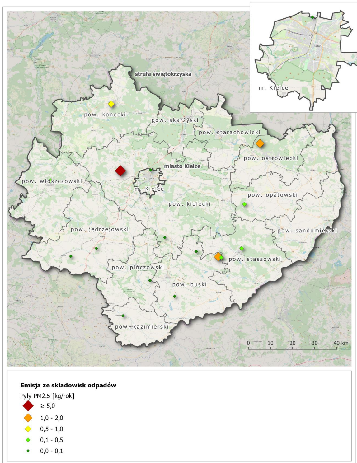
Rysunek 42. Emisja pyłu PM 2,5 ze składowisk odpadów 107
