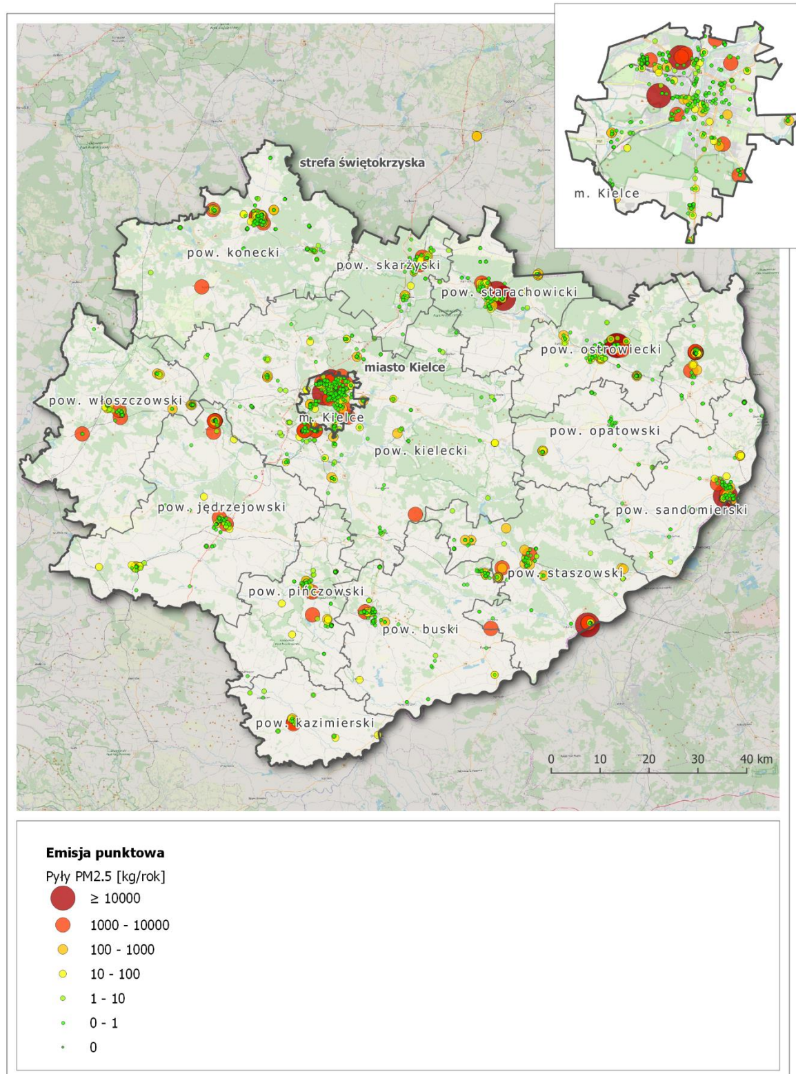
Rysunek 38. Emisja pyłu PM 2,5 ze źródeł przemysłowych i energetycznych 103
